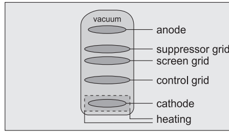
Fig. 4.6: Pentode
